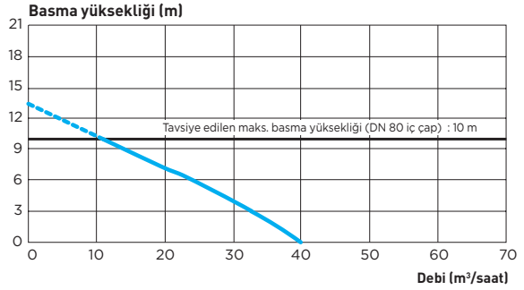
POMPA EĞRİSİ
